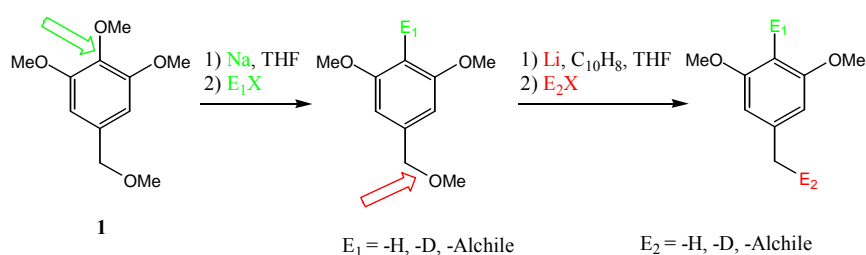
Schema 1. Scissione riduttiva del metil etere dell'alcool 3,4,5-trimetossibenzilico.
