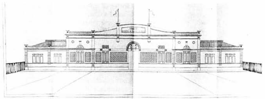
PROGETTO PER LA NUOVA SEDE DELLA SOCIETÀ DI EDUCAZIONE FISICA TORRES, IN SASSARI
