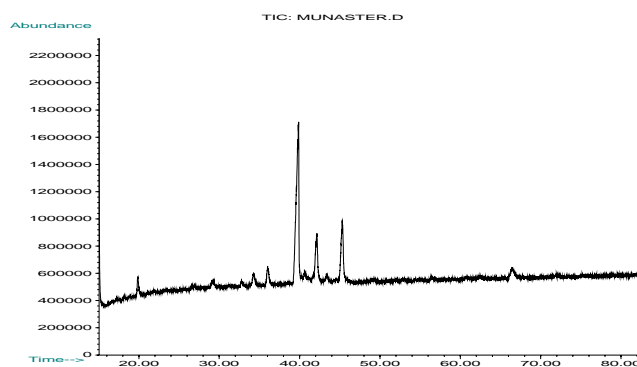
Tracciato gas cromatografico degli steroli da in saponificabile di Muña
