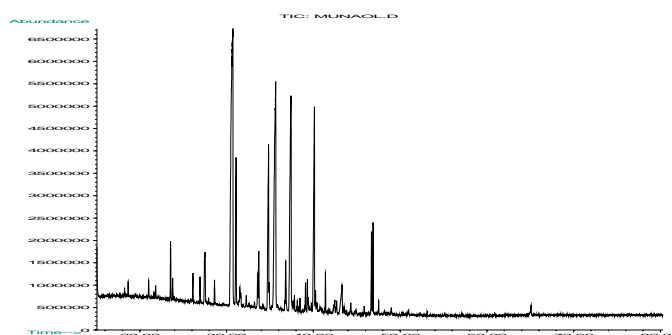
Tracciato gascromatografico dell'olio essenziale di Muña
