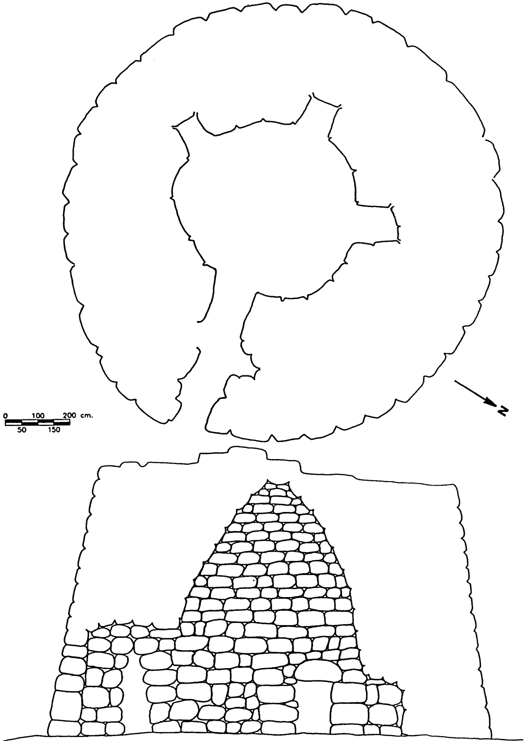
Figura 1. Nuraghe Lighei: planimetria e sezione.
