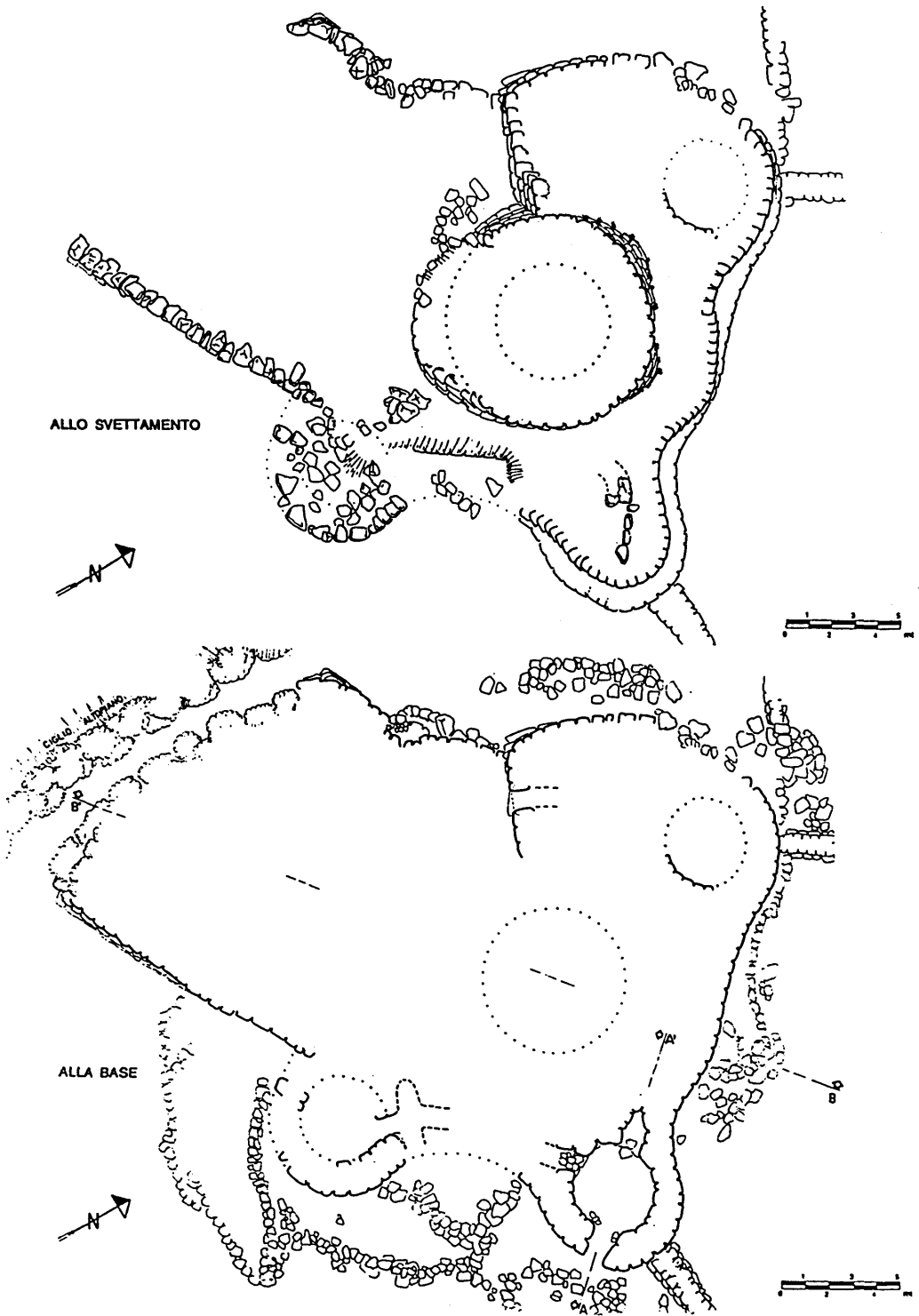
Figura 21. Nuraghe Iloi: planimetrie.
