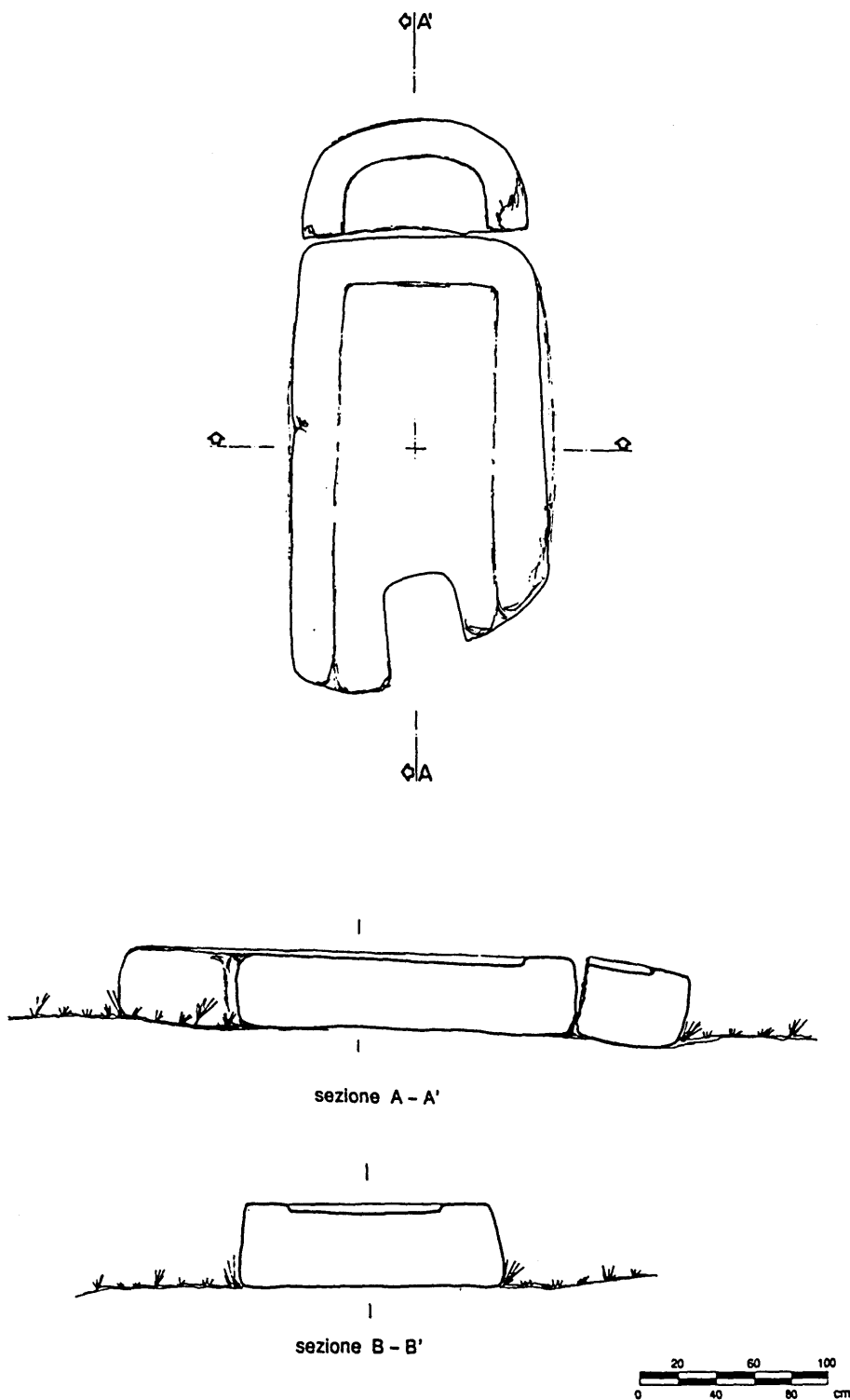
Figura 52. Stele di tomba di giganti di Mura-Aidomaggiore: prospetto, sezioni.
