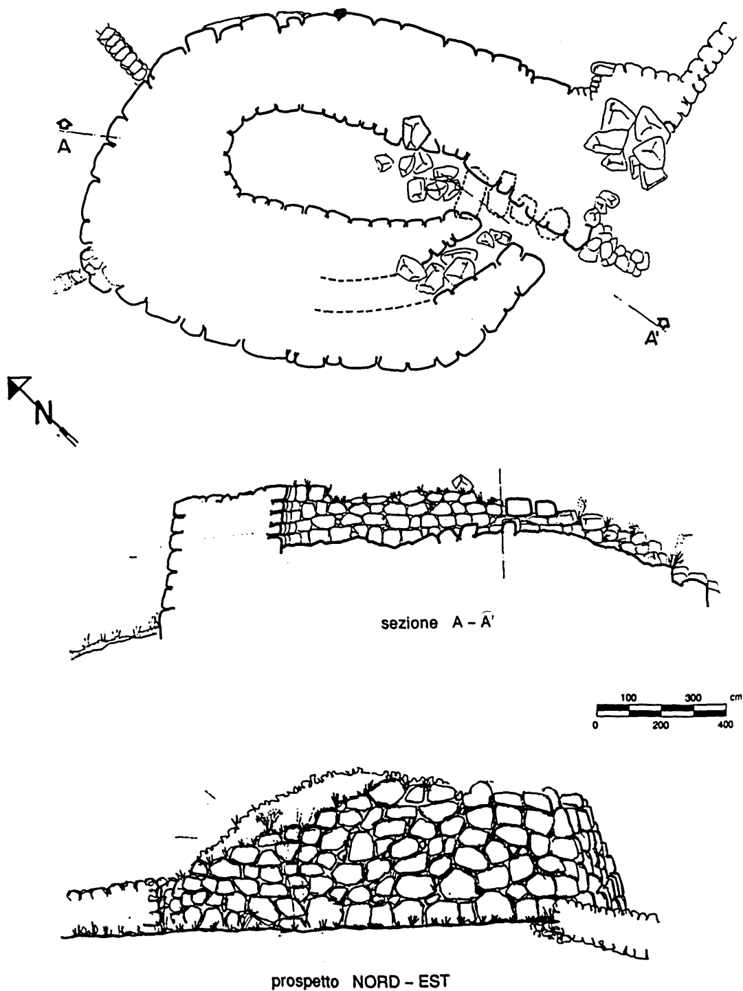
Figura 53. Nuraghe Padru Longu-Aidomaggiore: planimetria, sezione, prospetto.
