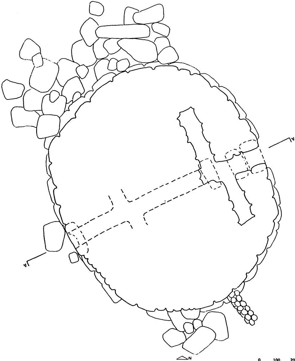
Figura 3. Nuraghe Ulinu: sezione e planimetria.
