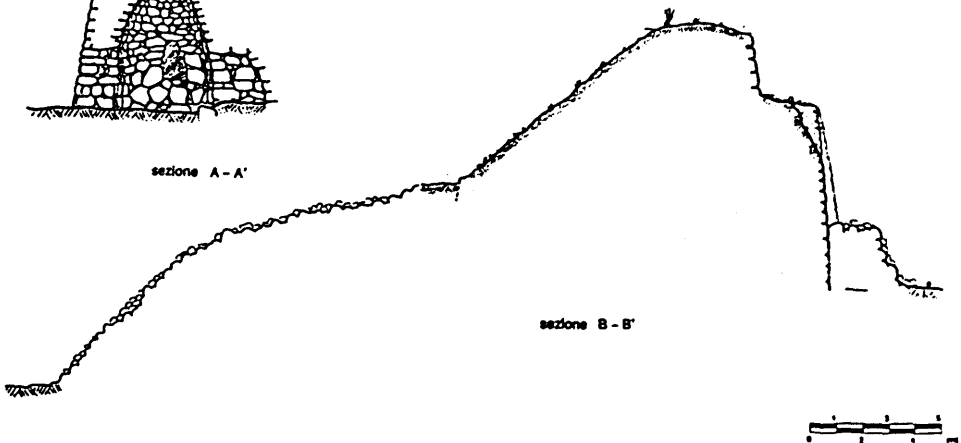
Figura 22. Nuraghe Iloi: prospetti, sezioni.
