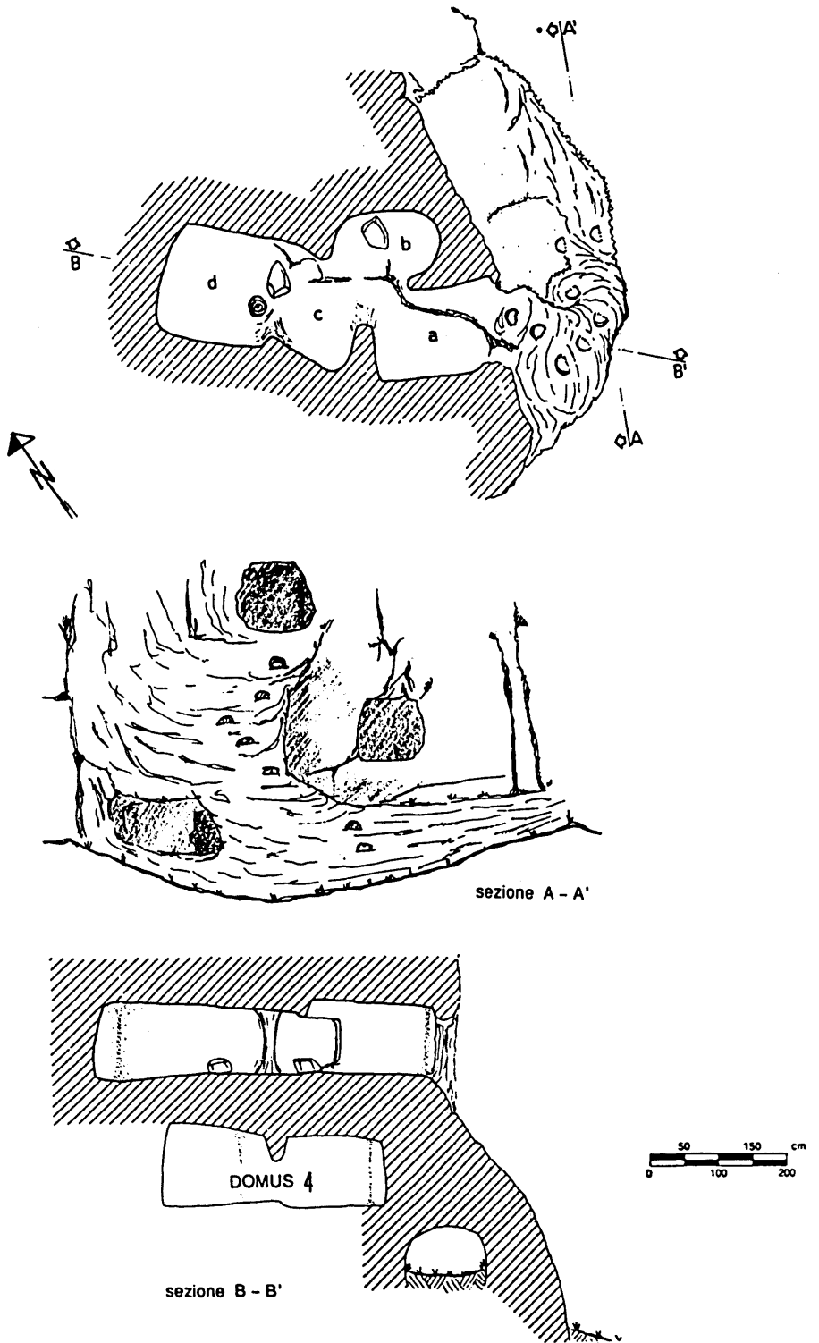
Figura 32. Ispituncas, domus de janas 5: planimetria, sezioni.
