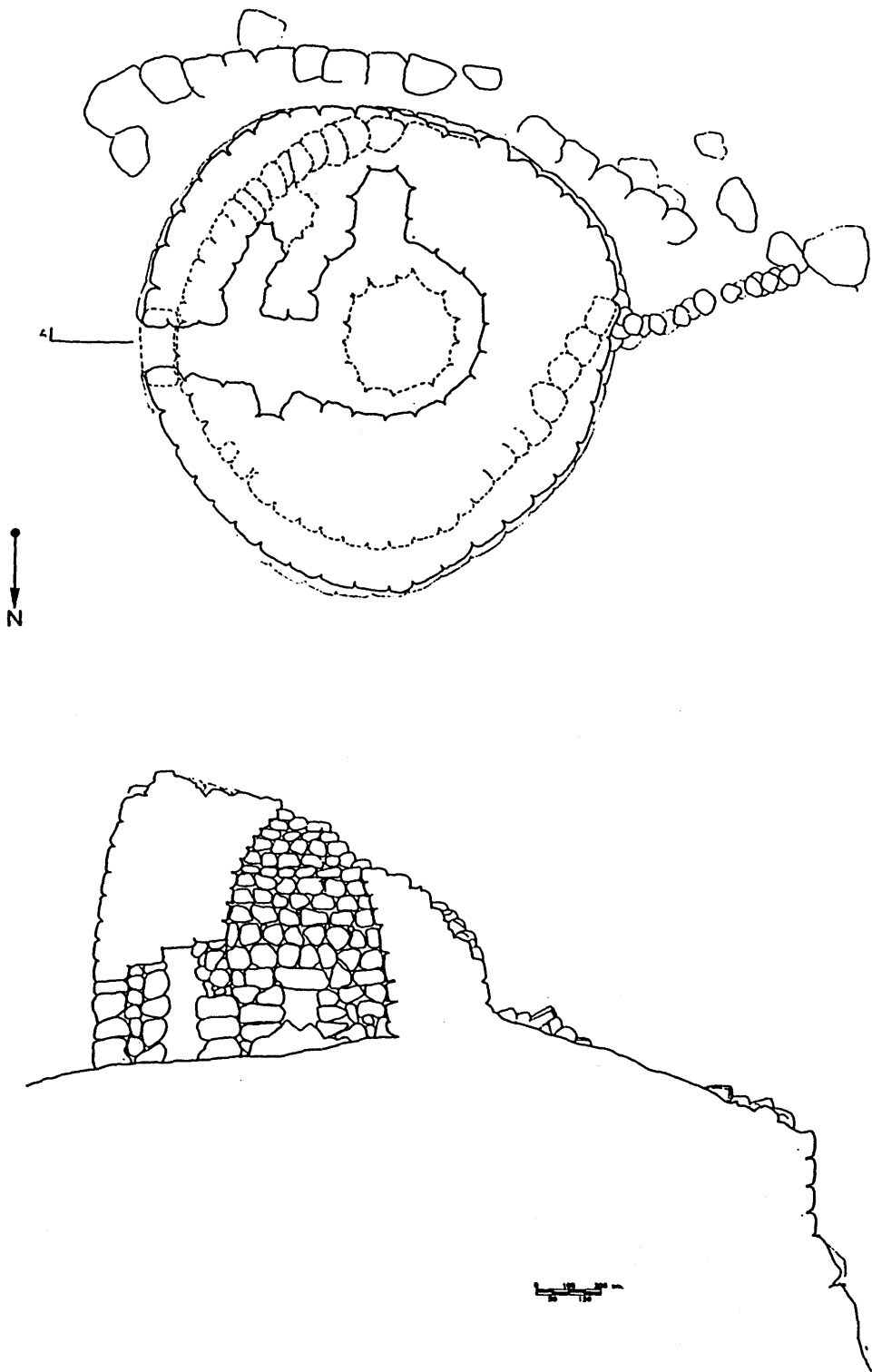
Figura 49. Nuraghe Talasoi: planimetria, sezione.
