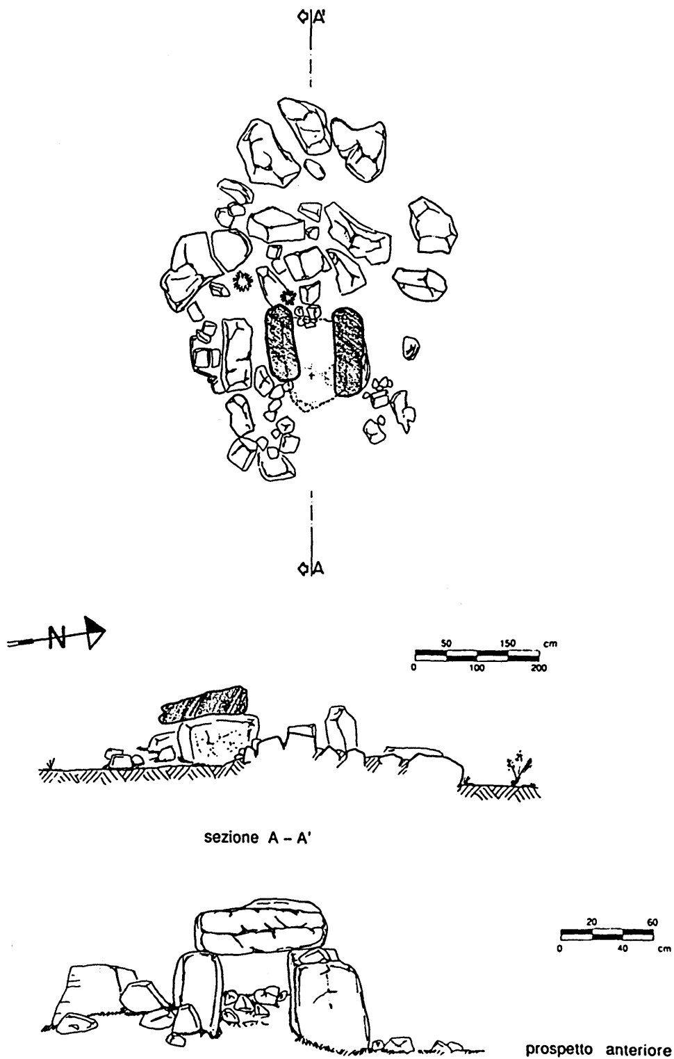
Figura 23. Dolmen Iloi: planimetria, sezione, prospetto.
