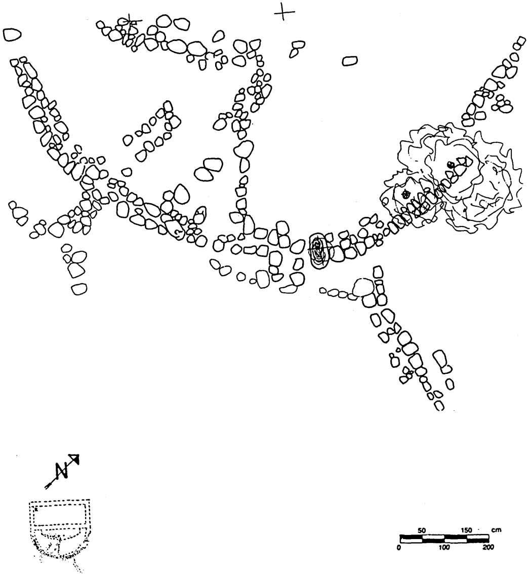
Figura 71. Copanno 9 di Serra Linto: planimetria.
