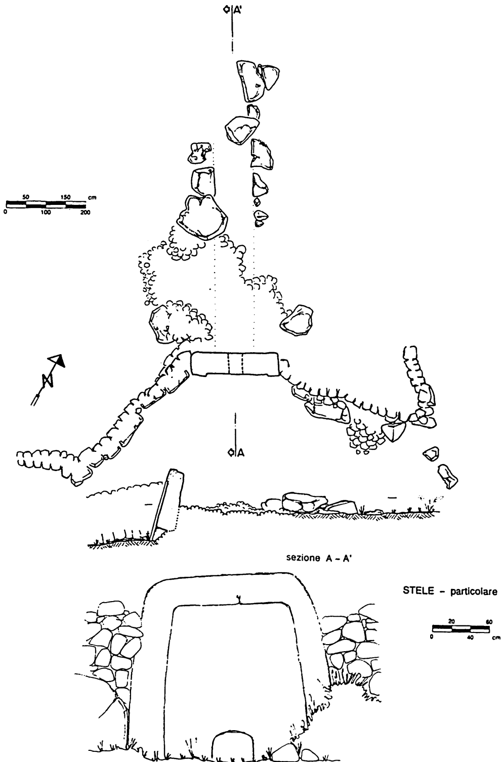
Figura 12. Tomba di giganti I di Scudu: planimetria, sezione, prospetto.
