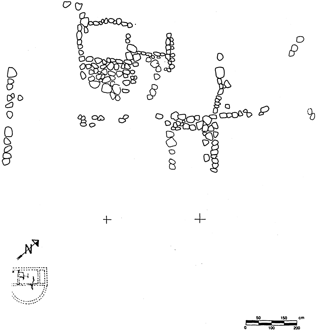
Figura 67. Capanna 5 di Serra Linta: planimetria.
