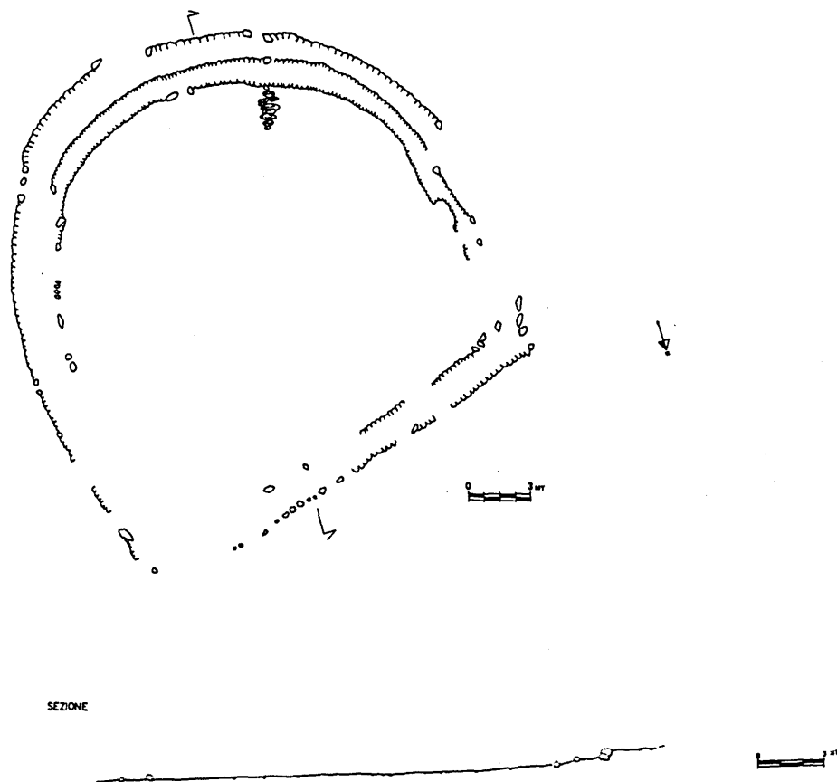
Figura 73. Struttura abitativa di Semo Linto: planimetria, sezione.
