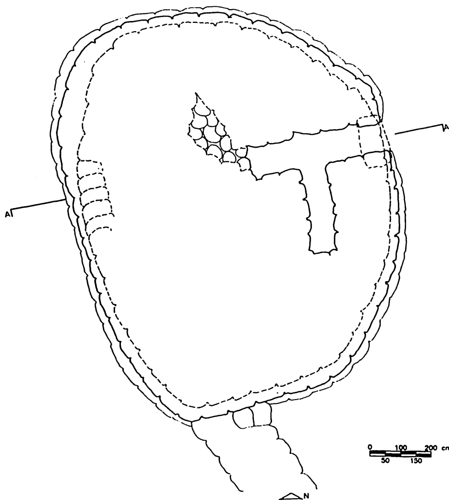
Figura 5. Nuraghe Scudu: sezione e planimetria.
