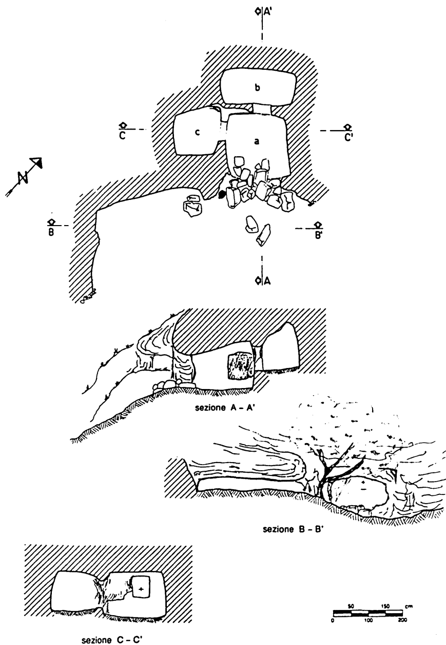
Figura 39. Ispiluncas, domus de janas 13: planimetria, sezioni.
