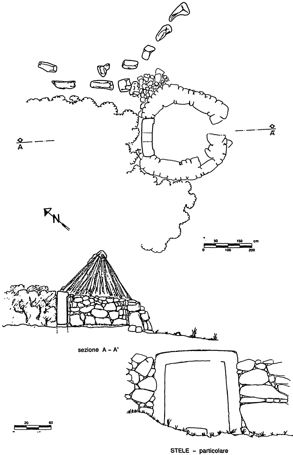
Figura 8. Tomba di giganti 2 di Uras-Aidomaggiore: planimetria, sezione, prospetto.
