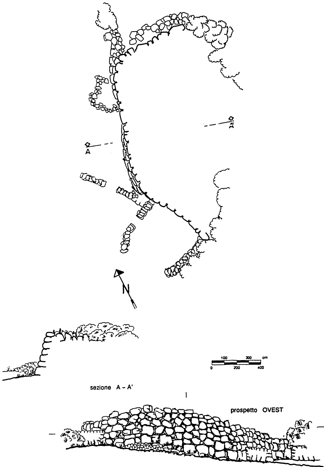
Figura 55. Nuraghe Mura-Aidomaggiore: planimetria, sezione, prospetto.
