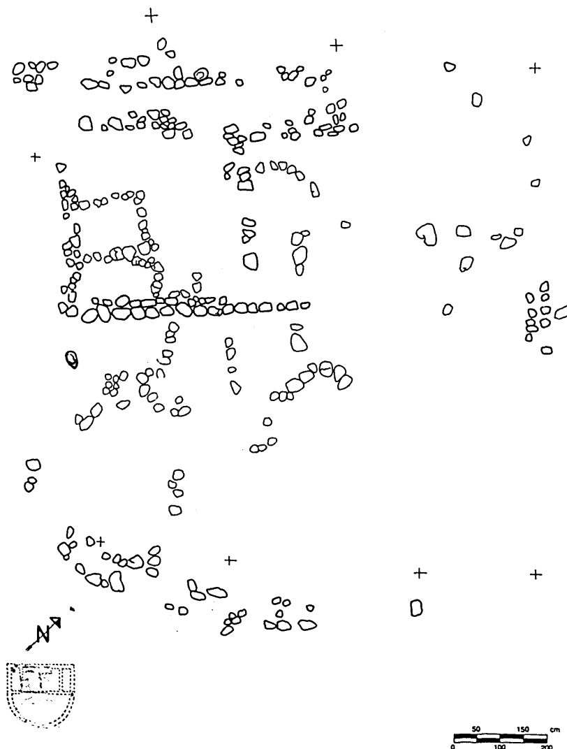
Figura 68. Capanna 6 di Serru Linta: planimetria.
