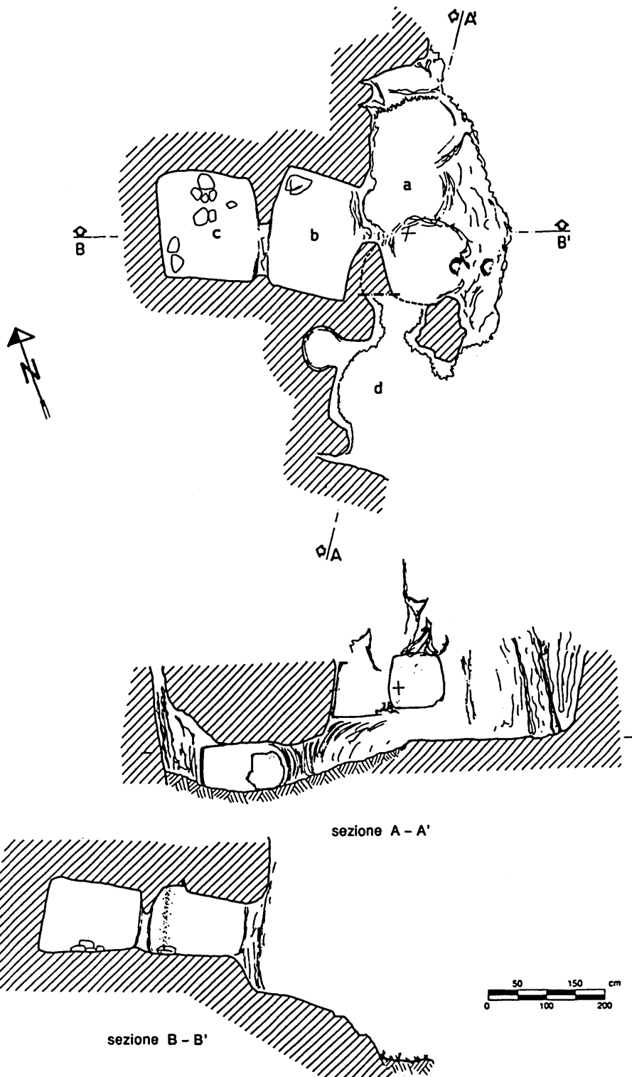
Figura 31. Ispiluncas, domus de janas 4: planimetria, sezioni.
