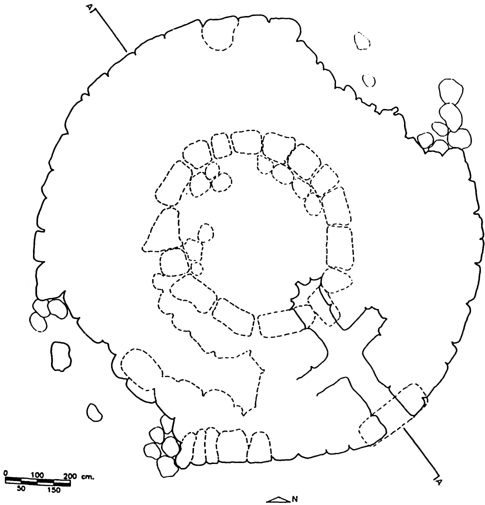
Figura 6. Nuraghe Puligone: sezione e planimetria.
