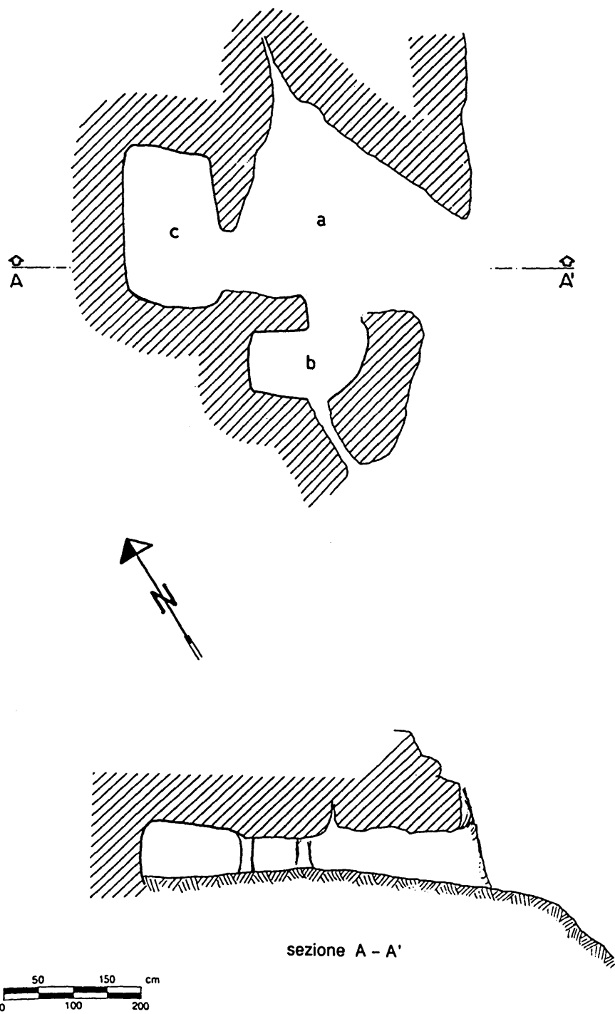
Figura 35. Ispiluncas, domus de janas 8: planimetria, sezione.
