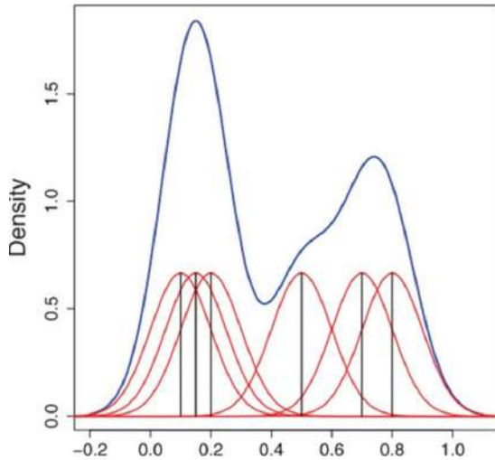
Fig. 8. Esempio geometrico-matematico della stima cumulata attraverso la KD [Chen 2017].
